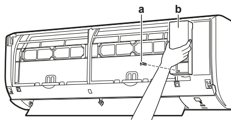
a Гвинт кришки для обслуговування
