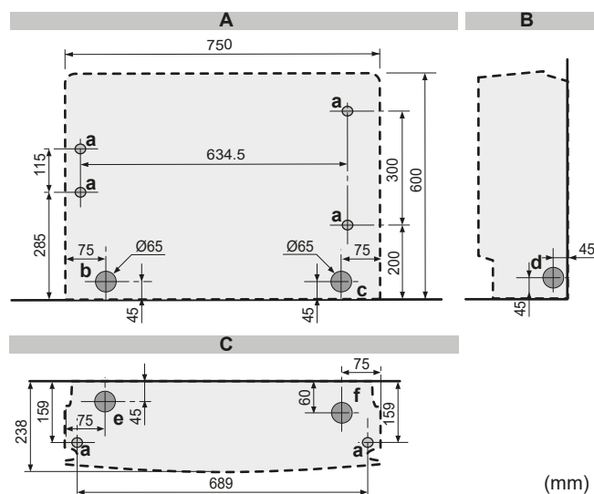
6-1 Креслення для встановлення внутрішнього блоку: Підлогове встановлення
