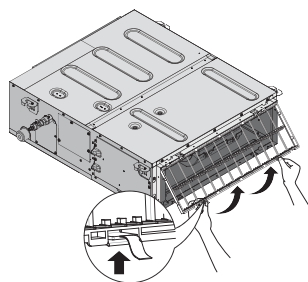
задній повітрозабірник
