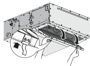
нижній повітрозабірник
