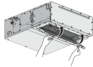
нижній повітрозабірник
