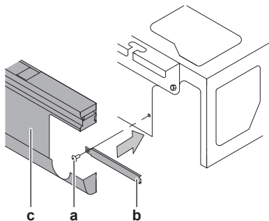
a Гвинт b Підсилювальна накладка c Декоративна бічна панель
