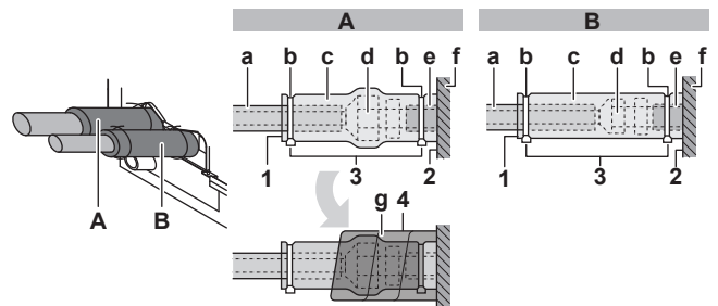
A Трубка газової фази B Трубка рідкої фази
