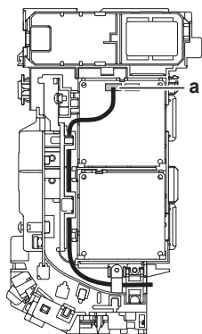
a Роз'єм S21
