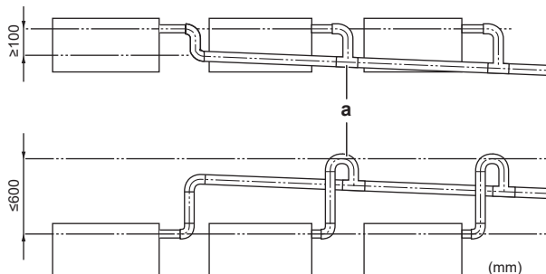
а Т-подібне з'єднання
