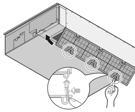
нижній повітрязабірник
