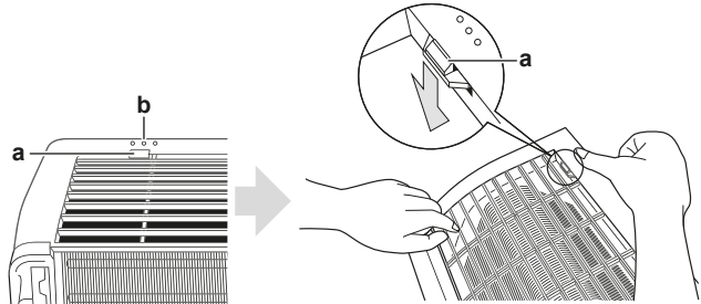
а Верхній гак b Символ з 3 колами
