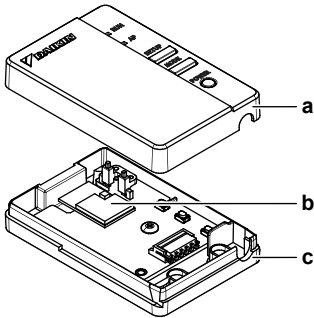
а Верхня частина корпусу б Плата адаптера бездротової локальної мережі с Нижня частина корпусу
