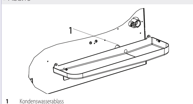
» Abb.15
