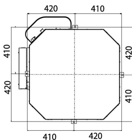
» Abb.5 FWH 06-07-08
