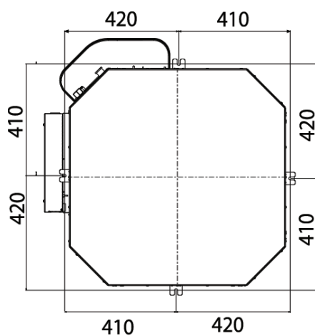
» Fig.5 06-07-08
