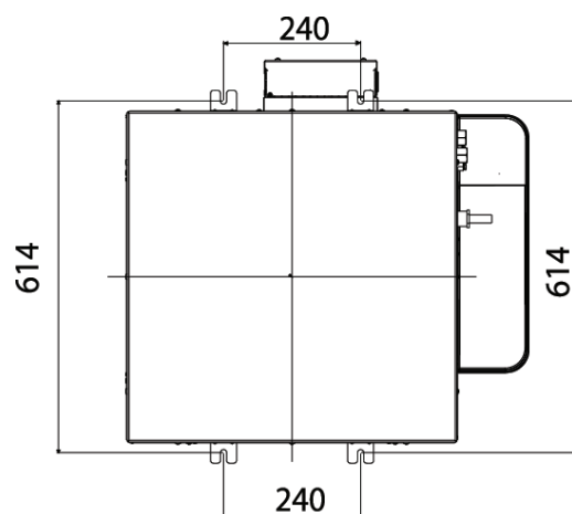
» Fig.4 FWH 02-03-04
