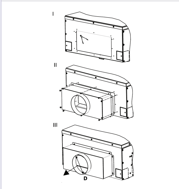
» PPA102A / 06A
